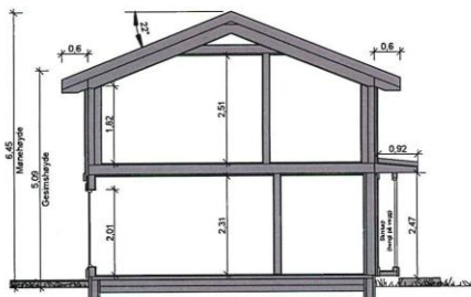
SNITT MOT LOFTSPLAN STUE OG SOV
