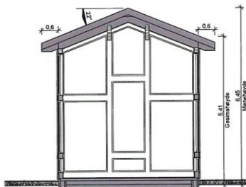
SNITT MOT STUE OG GALLERI LOFTSPLAN
