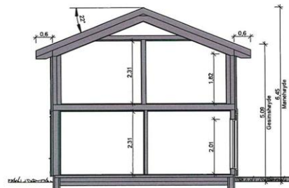
SNITT MOT LOFTSPLAN SOV 4 OG 5
