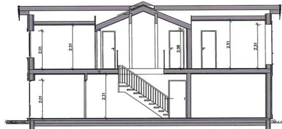
SNITT MOT BAD, BOD OG SOV 3 LOFTSPLAN
