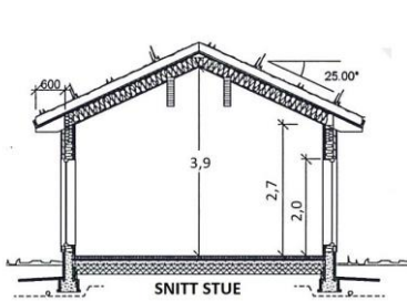
SNITT STUE
