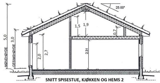
SNITT SPISESTUE, KJØKKEN OG HEMS 2
