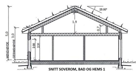
SNITT SOVEROM, BAD OG HEMS 1
